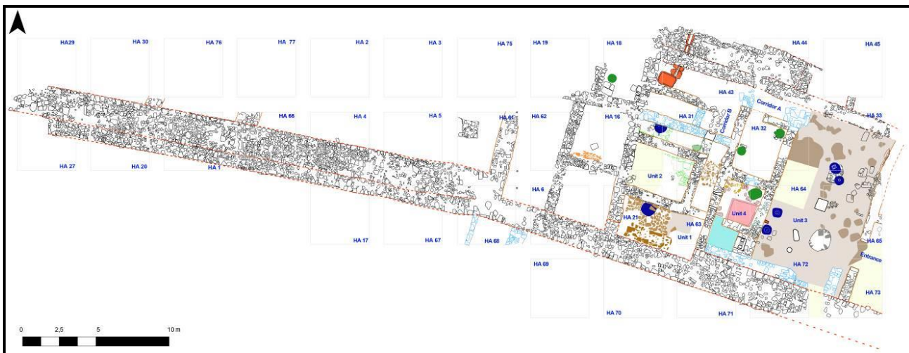
ΕΙΚ.12 Κάτοψη Συμπλέγματος Χατζηαπουλλά
