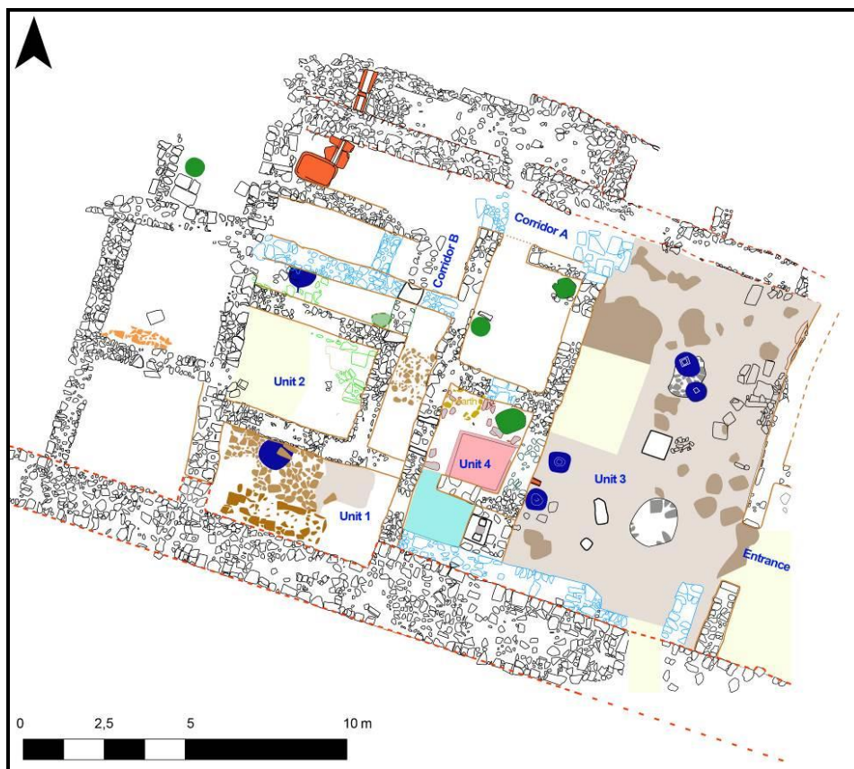
ΕΙΚ.13 Κάτοψη εργαστηριακών μονάδων
